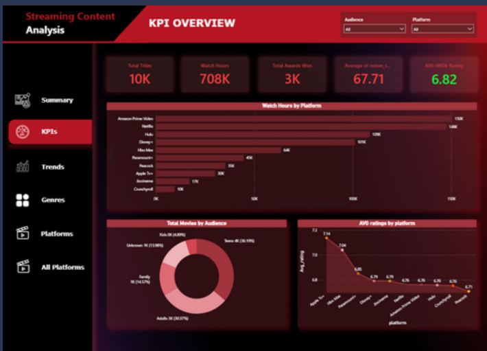
KPI Overview
